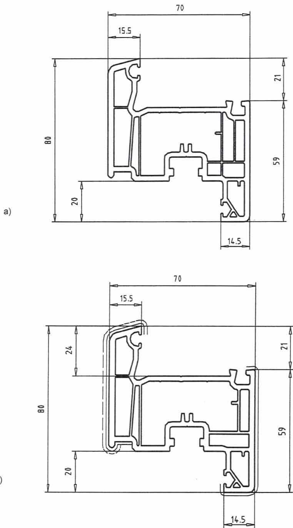
Rys. 15. Przekroje kształtowników z nieplastyfikowanego PVC
